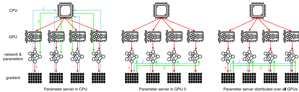
Fig. 13.7.3 Parameter synchronization strategies.
